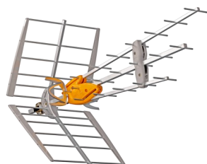
DAT BOSS - Gain 17 à 42dB max Réjection optimisée de la bande LTE à partir du canal 48 (698MHz)
